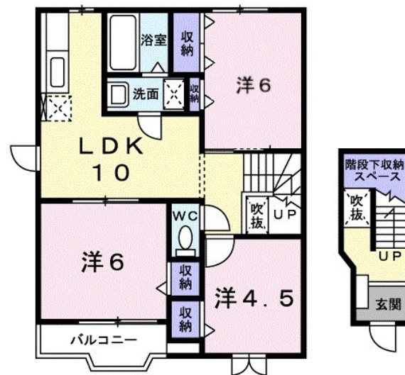
【間取り図】
