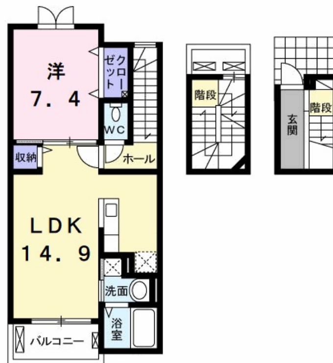
【間取り図】
