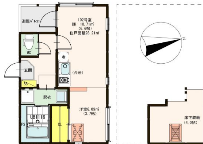
【間取り図】
