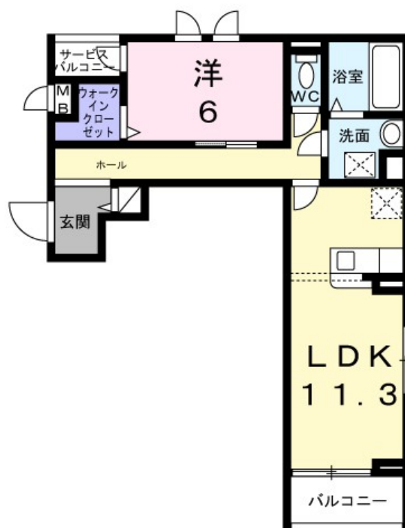
【間取り図】
