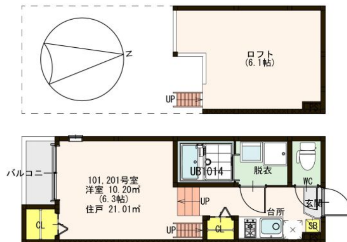
【間取り図】
