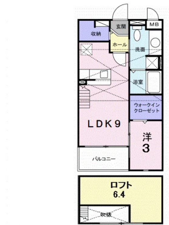
【間取り図】
