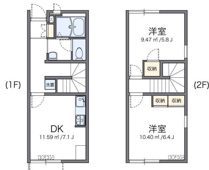
【間取り図】
