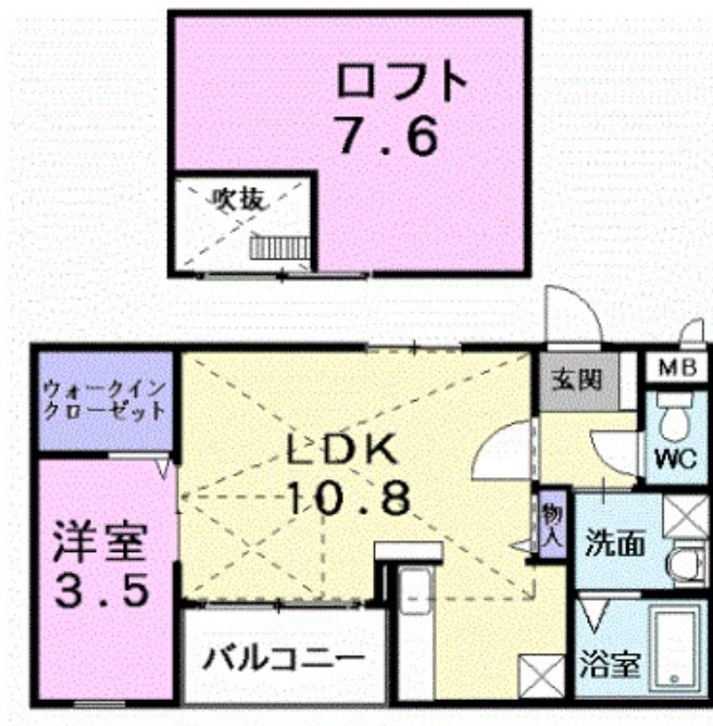
【間取り図】
